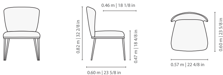
SIN BRAZO - BASE DE ACERO without arm - steel base | sin brazo - base de acero
