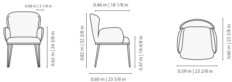
CON BRAZO - BASE DE ACERO with arm - steel base
